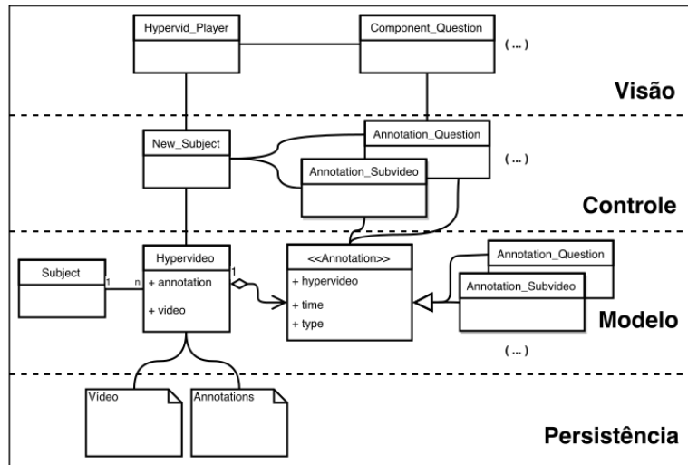
Figura 10 – Arquitetura planejada para integração com Hipervídeos. Fonte: Própria.
