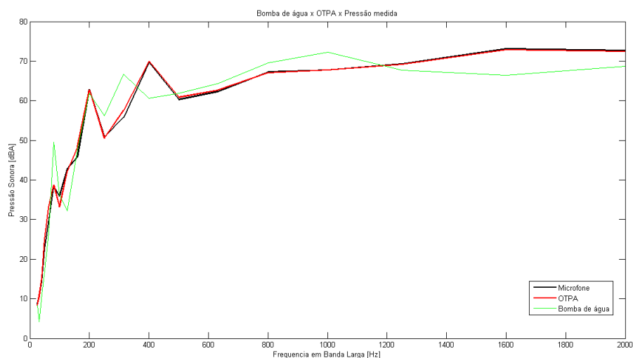
Figura 59: Comparação gráfica entre, a contribuição individual da bomba d'água, o nível de ruído calculado e o nível de ruído medido
