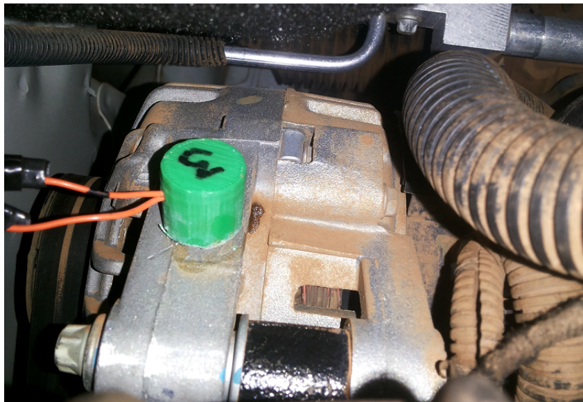
Figura 44: Posição do acelerômetro no caminho associado ao alternador
