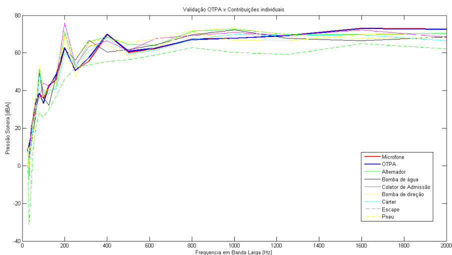
Figura 57: Comparação gráfica entre, as todas contribuições individuais, o NPS calculado e o NPS medido
