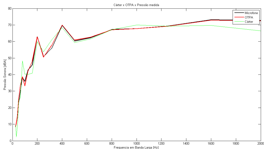
Figura 62: Comparação gráfica entre, a contribuição individual do cárter, o nível de ruído calculado e o nível de ruído medido
