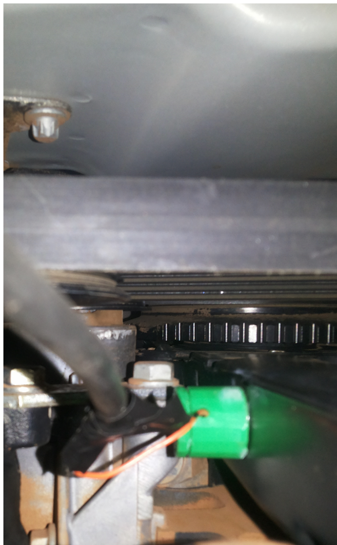
Figura 41: Posição do acelerômetro no caminho associado a bomba d'agua
